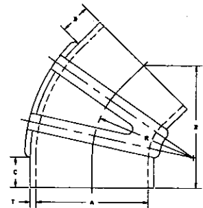
45° Elbow
