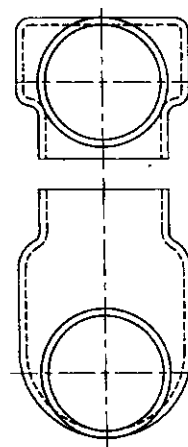
90° Cobra Elbow
