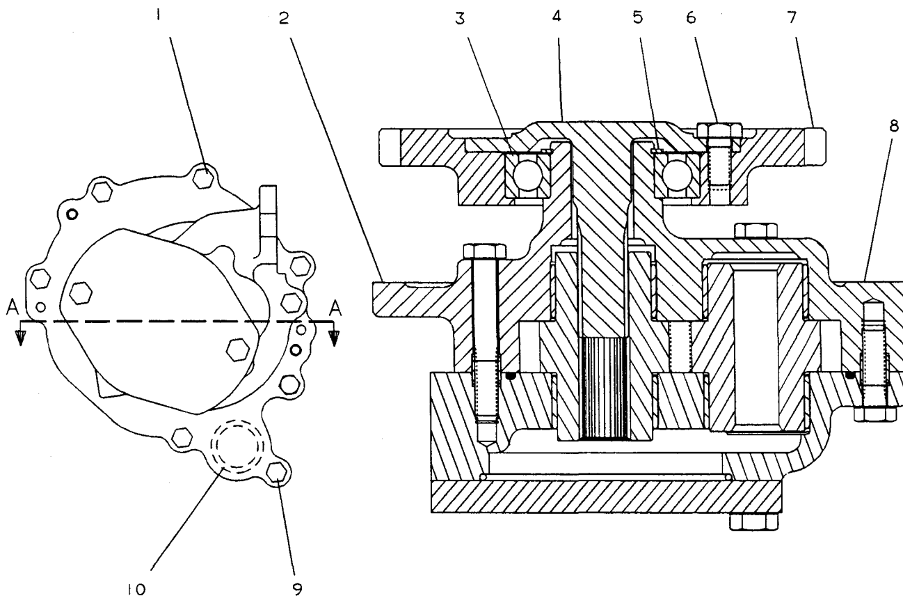
SECTION A-A
