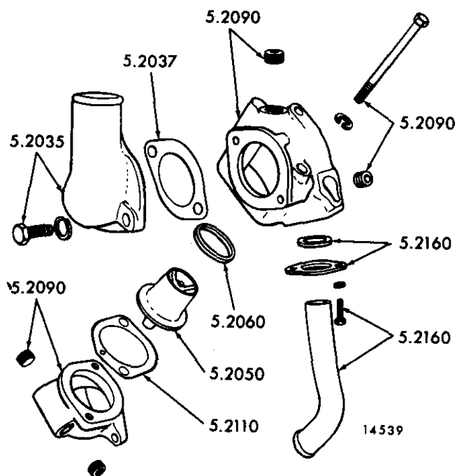
FIG. 3A THERMOSTAT (V-Models)
