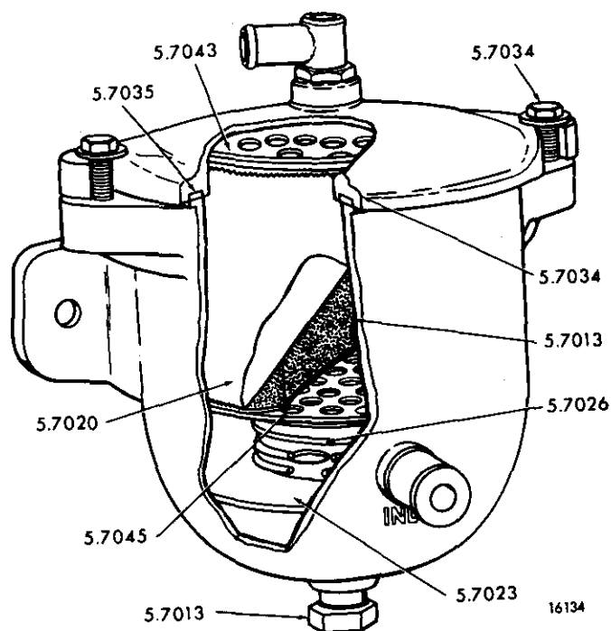
FIG. 9A WATER FILTER (Perry)
