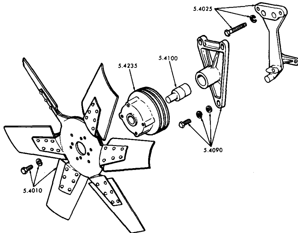
FIG. 4A FAN SHAFT & PULLEY
