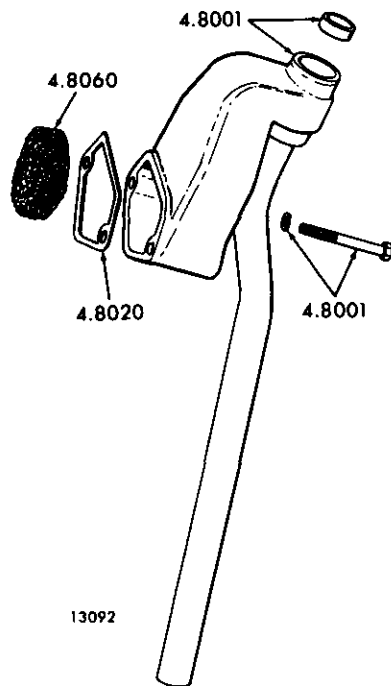
FIG. 8A BREATHER
