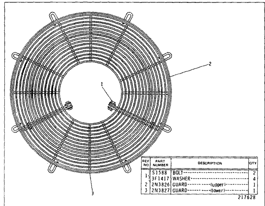
7N8935 FAN GUARD GROUP
