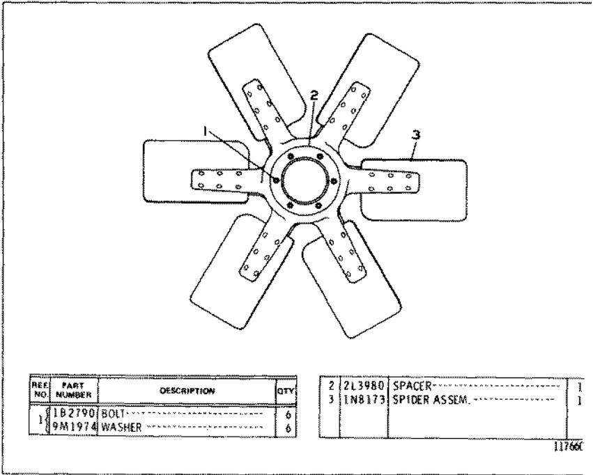
4N4684 BLOWER FAN GROUP—26 Inch (660 mm)
