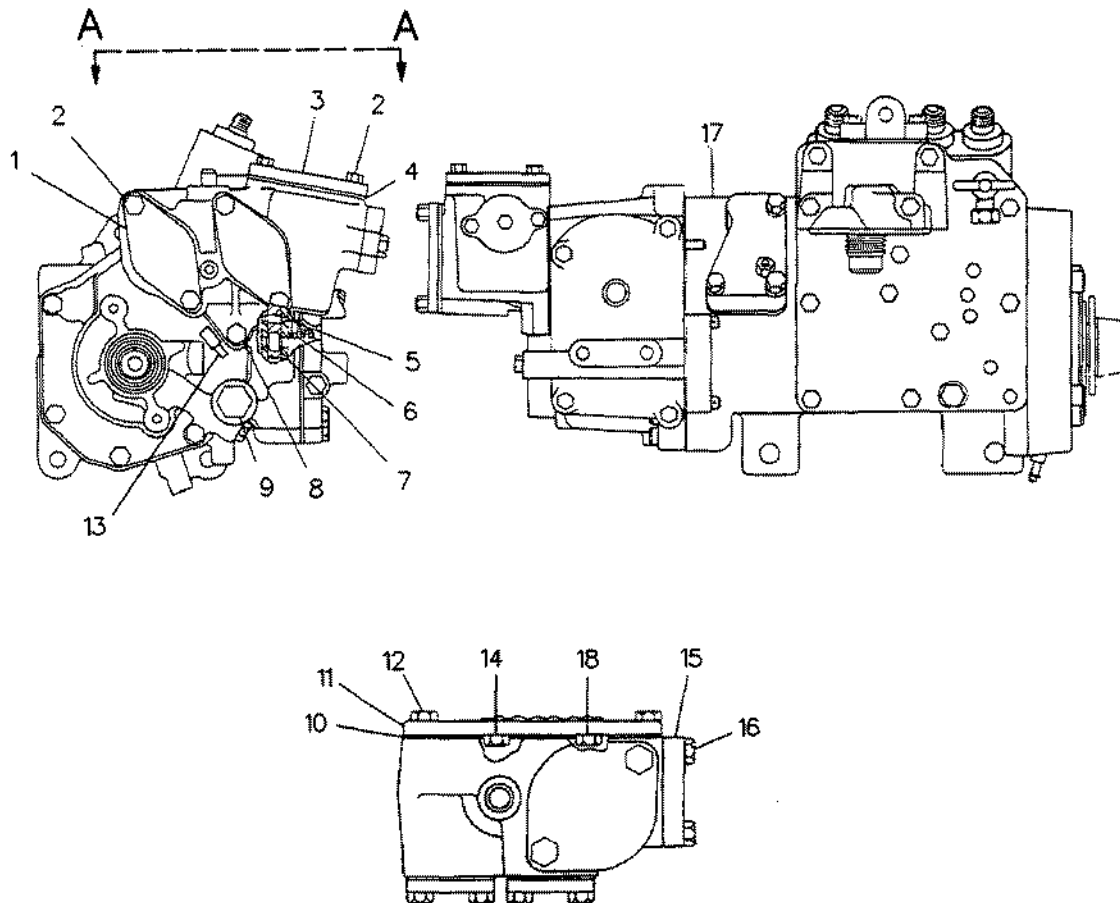
VIEW A-A
