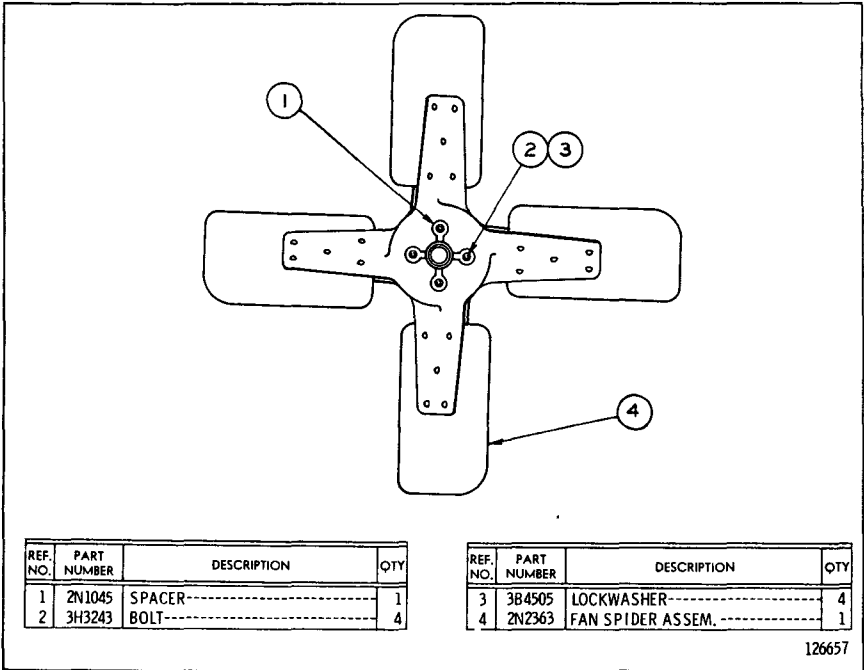
2N2458 SUCTION FAN GROUP—22" Diameter
