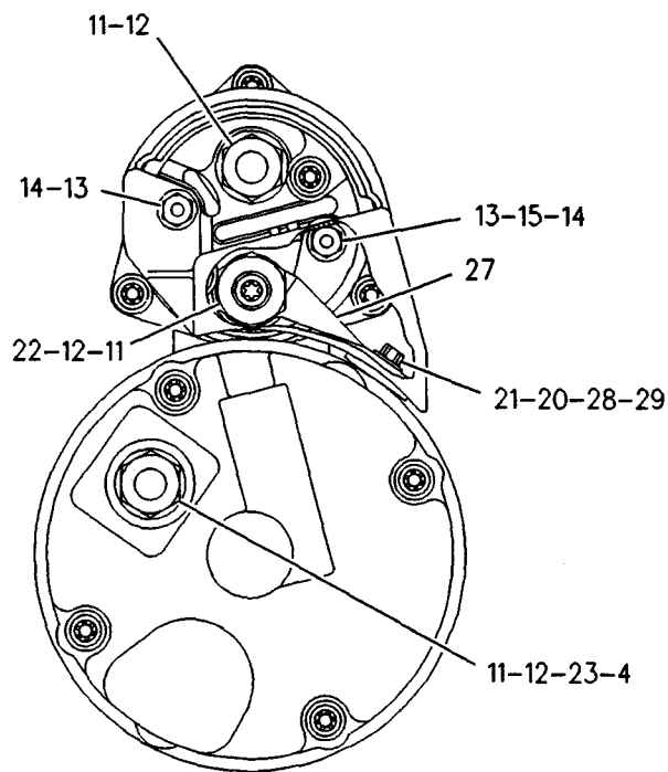
VIEW A-A
