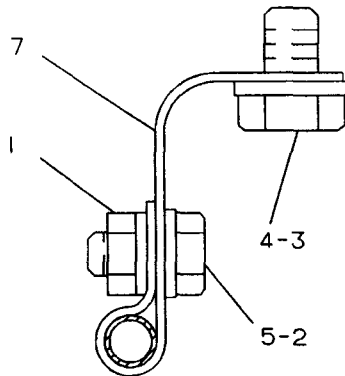
VIEW A-A
