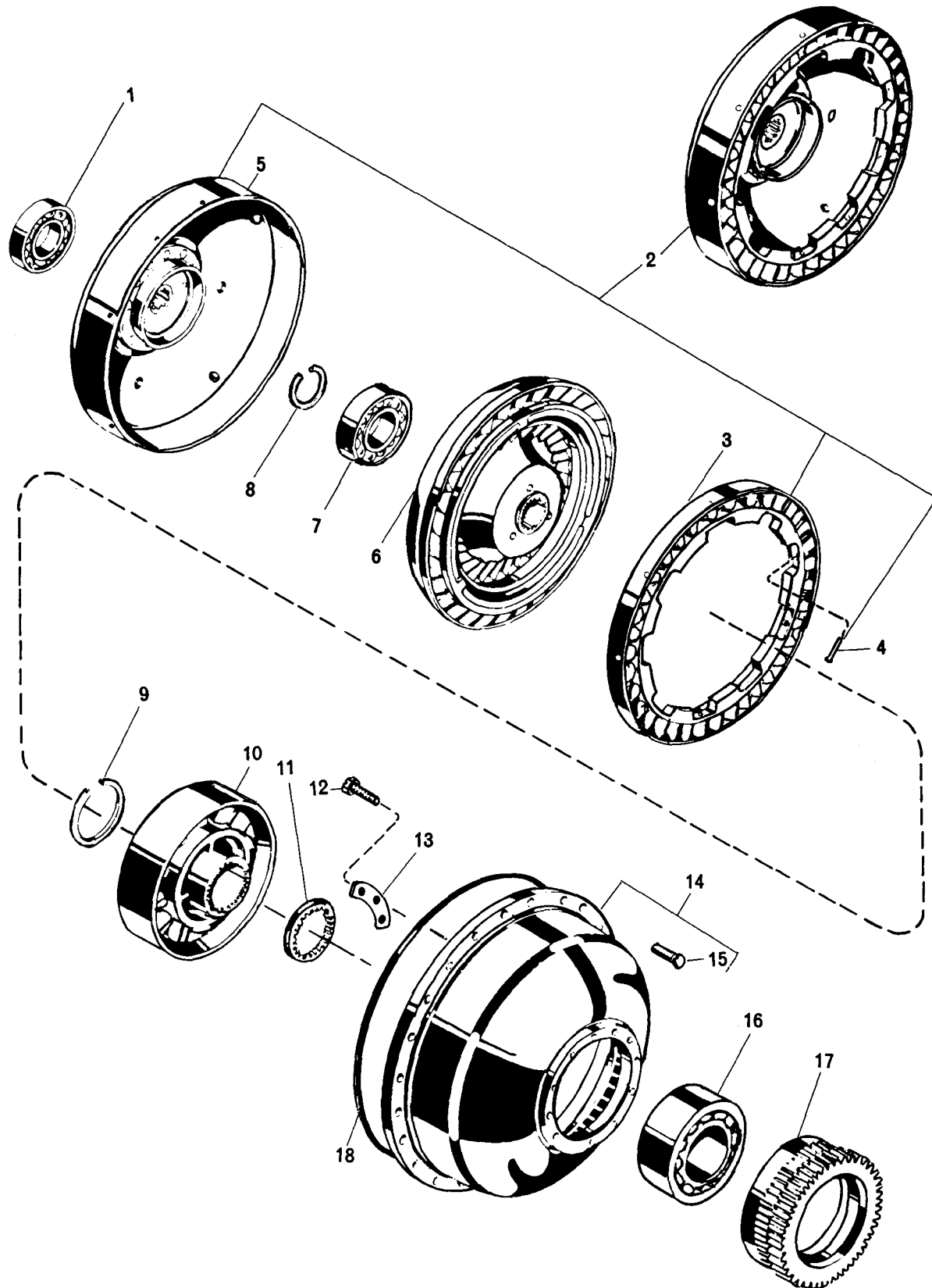
FIG. 4. TORQUE CONVERTER
