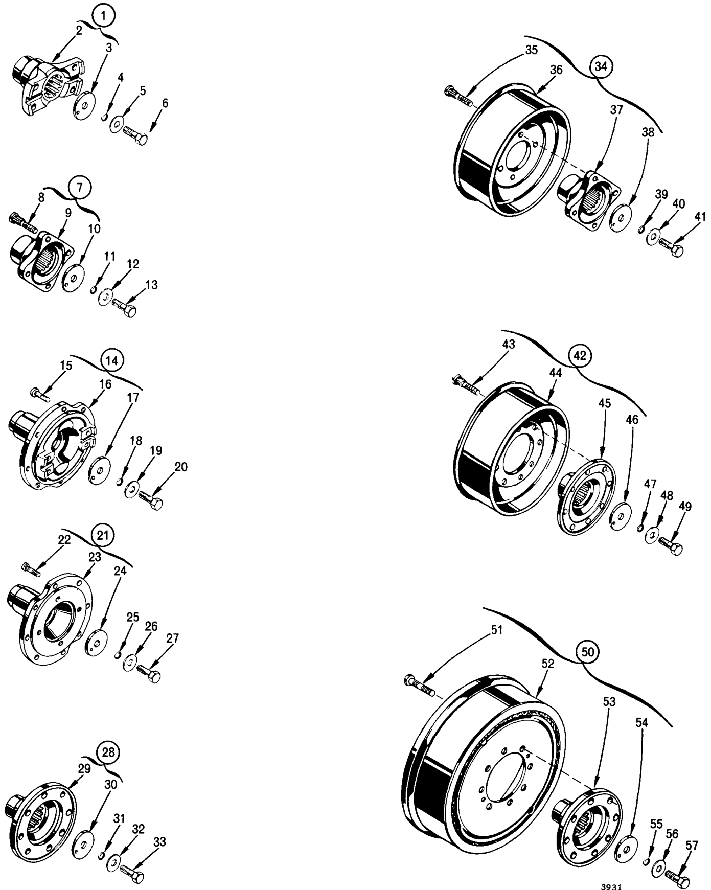
FIG. 13 FLANGE
