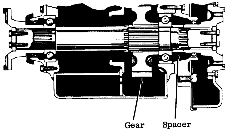
Fig. 1. Optional configuration
