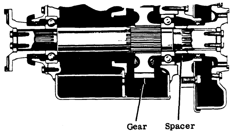
Fig. 1. Optional configuration
