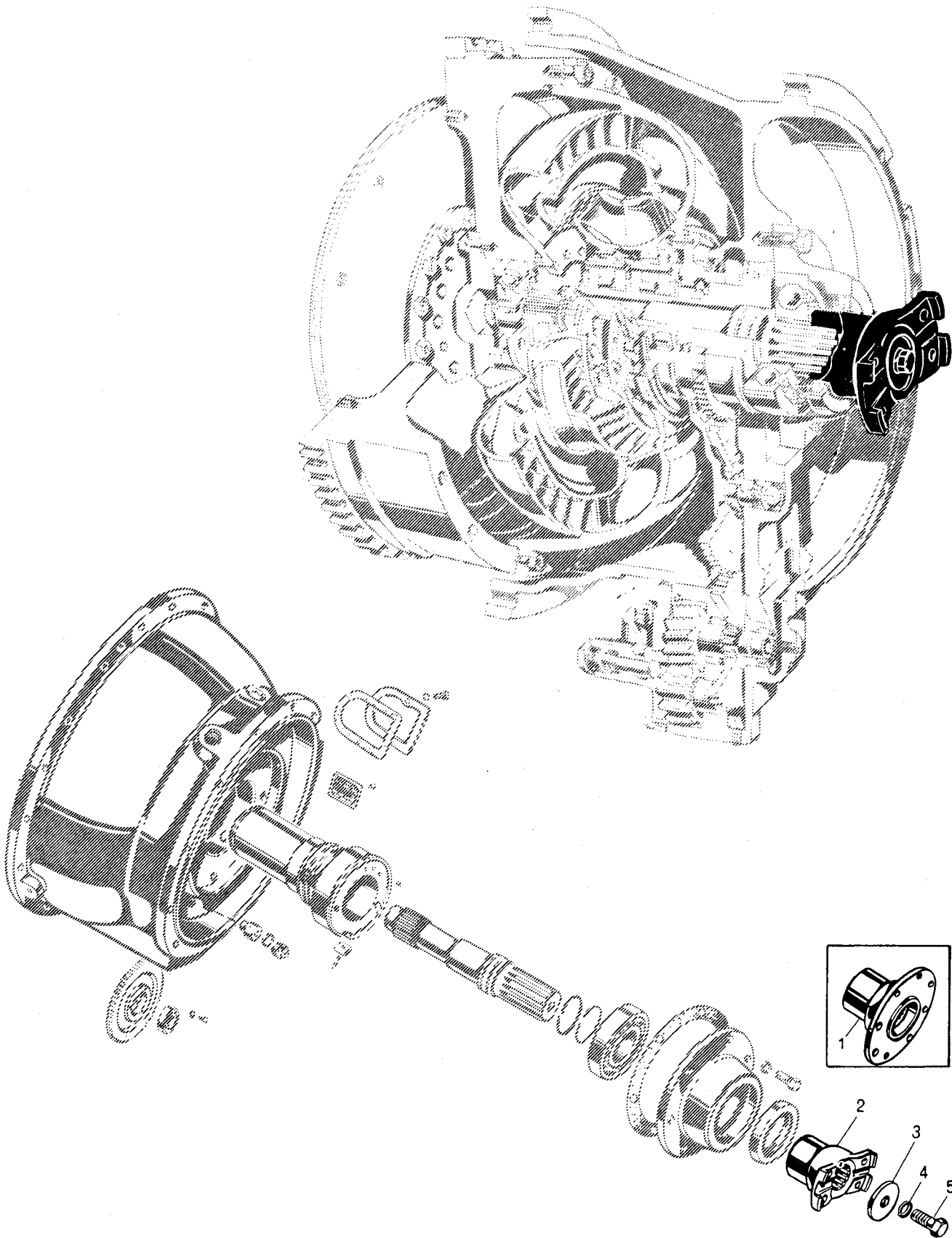
FIG. 8. FLANGE
