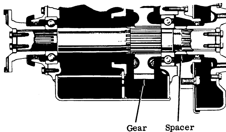
Fig. 1. Optional configuration
