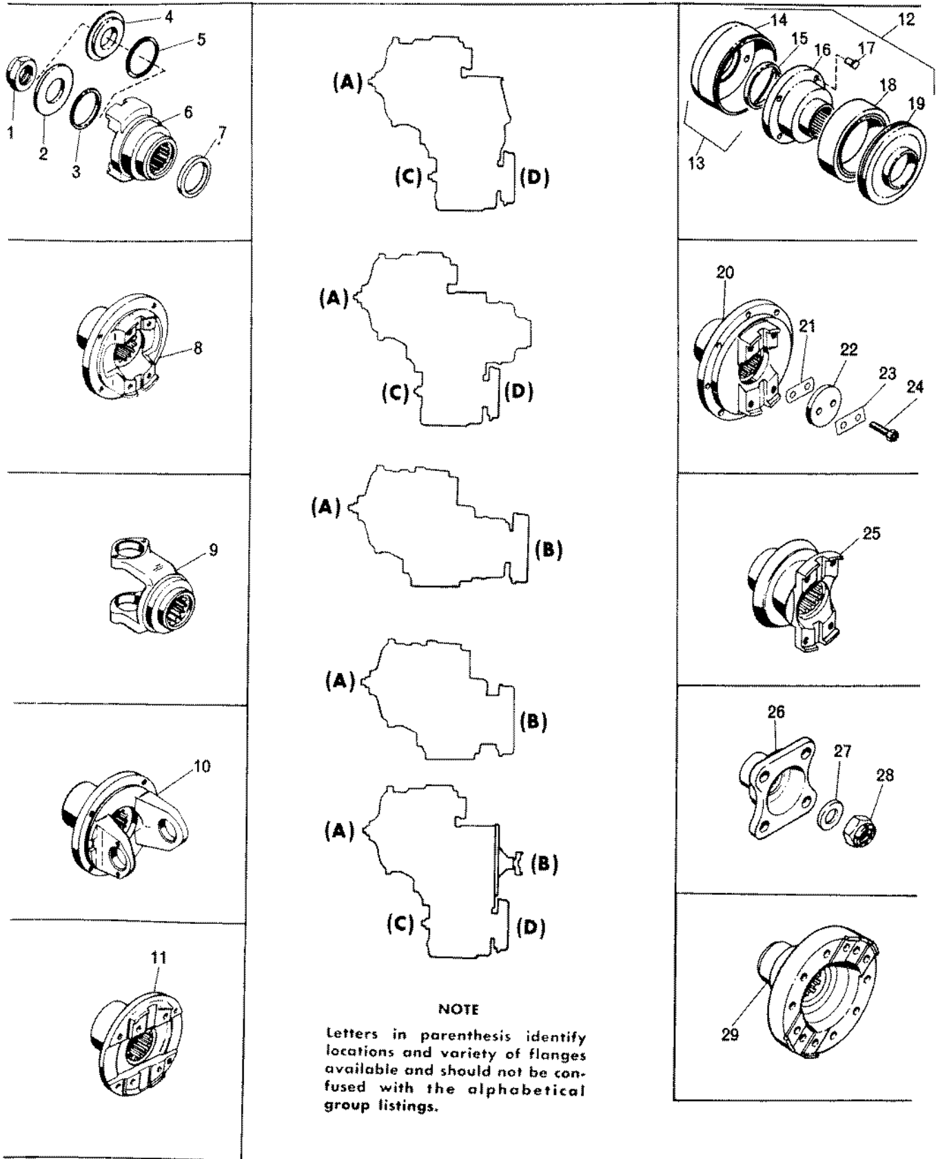
FIG. 1. FLANGE
