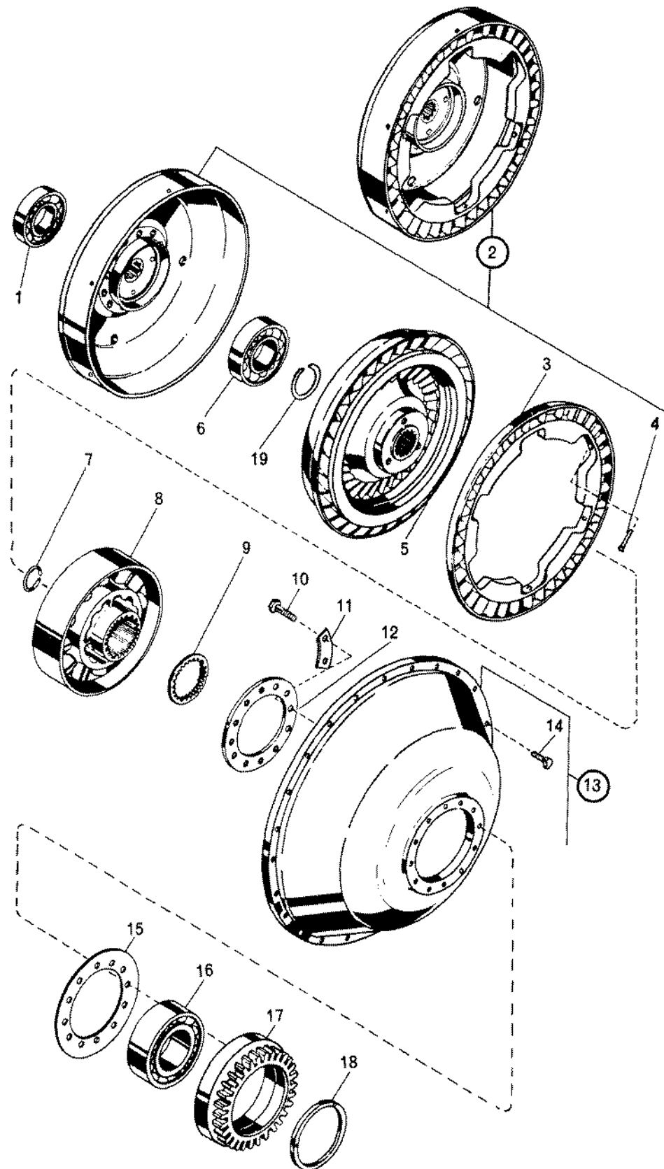
FIG. 4. TORQUE CONVERTER
